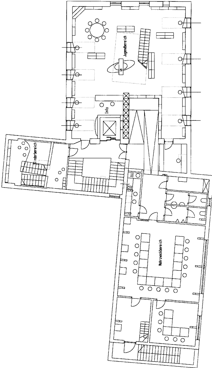
5 St. Michael/Eppan: Grundriß 2. Obergeschoß
