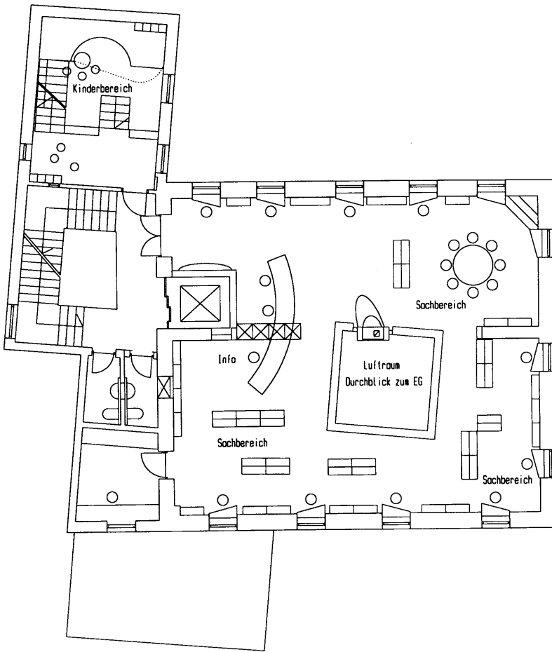
1. Obergeschoss
